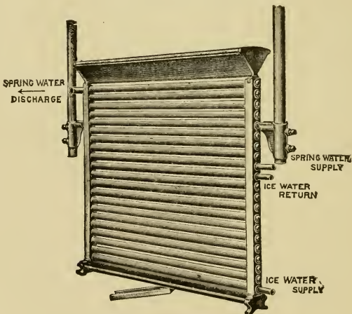
Tubular Cooler.
